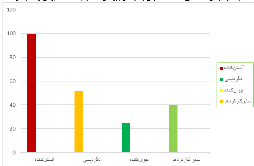
نمودار ۳- بسامد کارکردهای سیب در داستان‌های ایرانی و اروپایی
